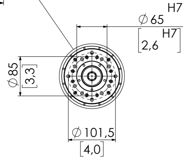
DETTAGLIO A SCALA 1 : 5
